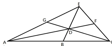
图 1.10: 定理1.2.8的证明
