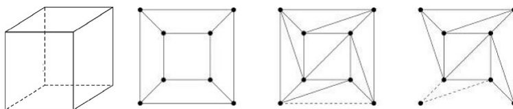
图 6.23: 欧拉多面体公式的证明
