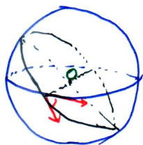
图 2.10: 球面的角
