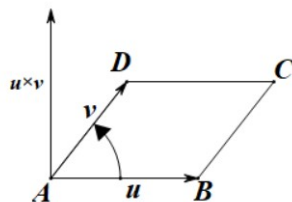
图 2.8: 外积
