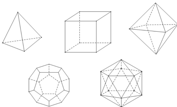
图 6.8: 五种正多面体
