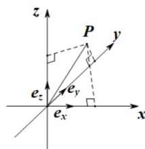
图 2.7: 右手系
