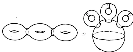
图 6.12: 亏格为 3 的曲面
