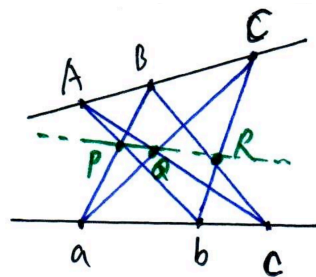
图 5.5: 帕普斯定理
