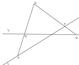
图 5.12: 透视投影
