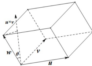
图 2.9: 平行六面体
