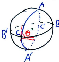
图 2.11: 球面二角形
