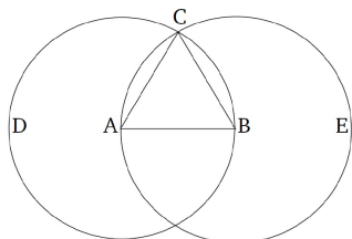
图 1.7: 《几何原本》命题 1
