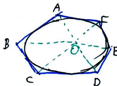
图 5.11: 对偶帕斯卡定理
