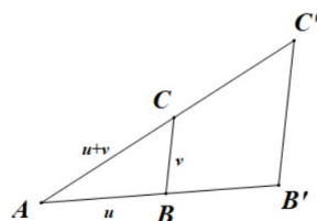
图 2.4: 相似三角形
