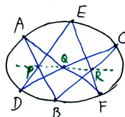
图 5.6: 帕斯卡定理
