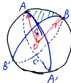
图 2.12: 球面三角形
