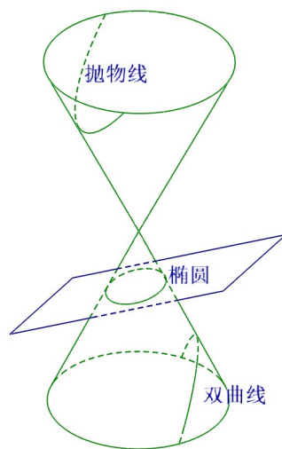
图 1.6: 圆锥曲线
