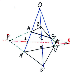
图 5.7: 德萨格定理
