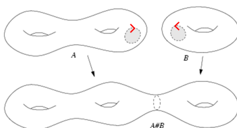
图 6.14: 连通和
