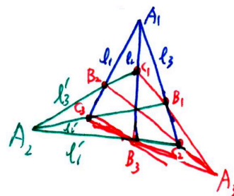
图 5.9: 对偶帕普斯定理
