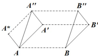
图 2.2: 平移的复合
