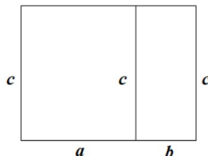
图 1.5: 加法分配率
