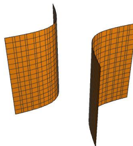
图 3.9: 双曲柱面
