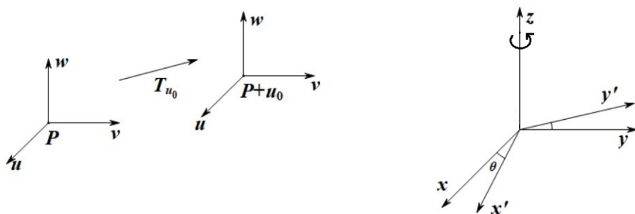
图 3.13: 平移与旋转
