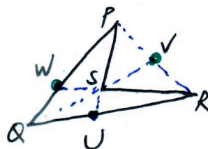
图 5.8: 完全四点形
