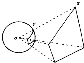
图 6.9: 多面体往球面的中心投影
