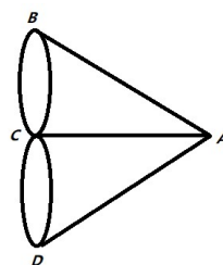
图 6.20: 欧拉转化后的问题
