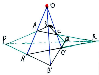
图 5.10: 对偶德萨格定理
