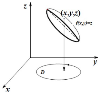
图 3.2: 曲面
