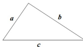
图 1.3: 勾股定理
