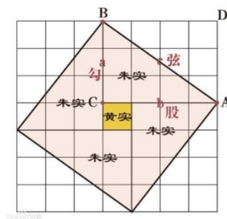
图 1.12: 弦图
